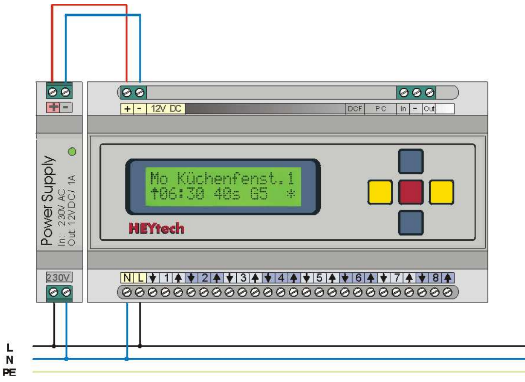
Rolladensteuerung, Modulsteuerung für Hutschienenmontage: Anschlussbild - Netzteil, Steuerung
