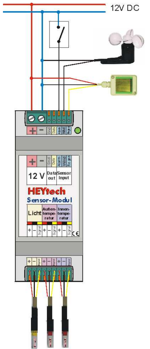
Anschlussbild Rolladensteuerung bzw. Wintergartensteuerung: Sensor-Modul und Sensoren
