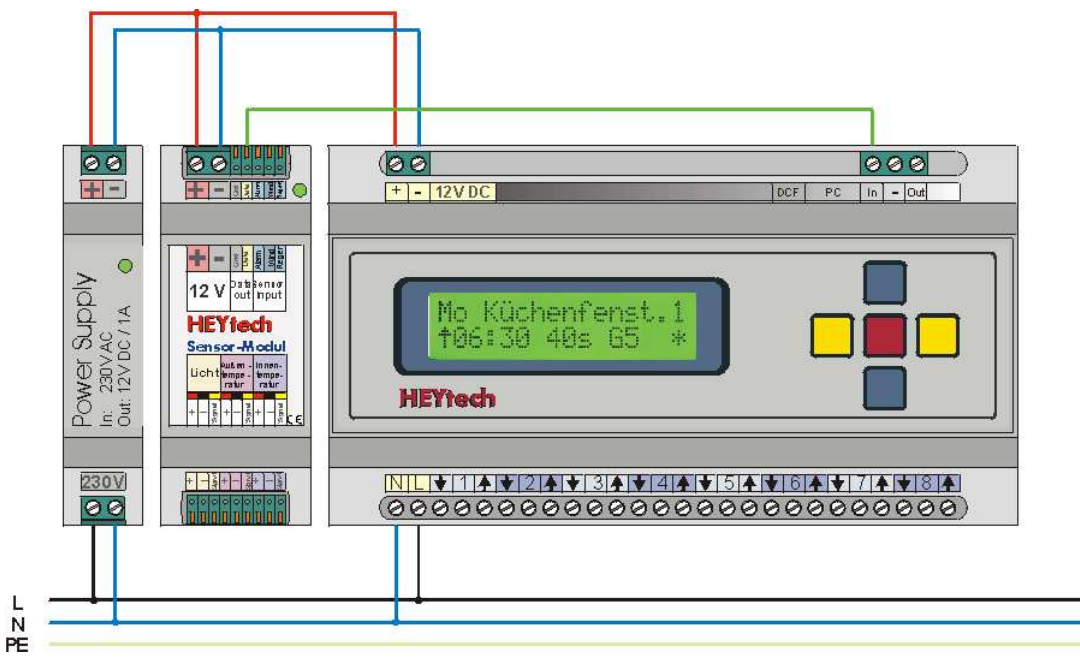
Rolladensteuerung, Modulsteuerung: Anschlussbild Netzteil, Sensor-Modul, Steuerung
