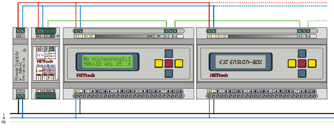
Rolladensteuerung, Modulsteuerung: Anschlussbild Netzteil, Sensor-Modul, Steuerung, Extension-Box
