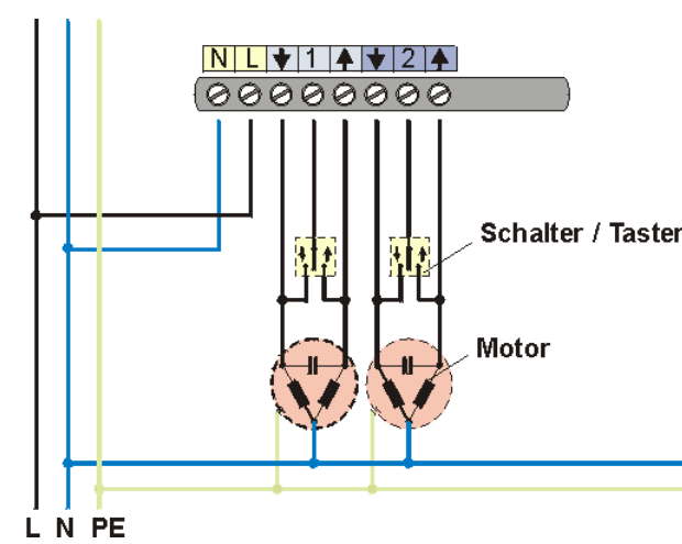
Detailbild Rolladensteuerung: Anschluss der Motoren und Bedienschalter
